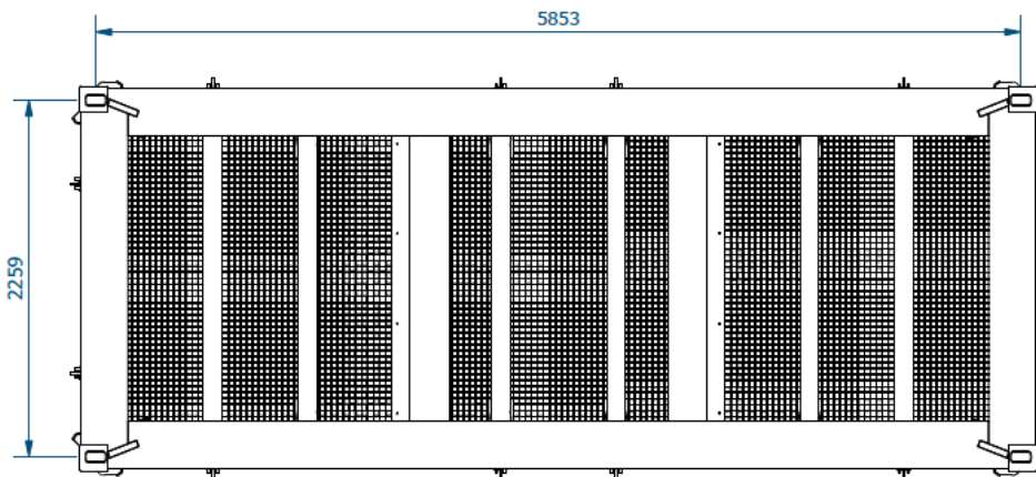
VIEW3 ( 1 : 40 )
