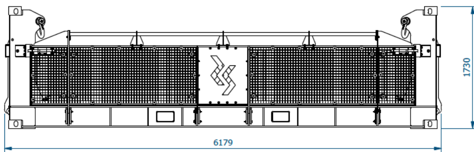
VIEW3 ( 1 : 40 )
